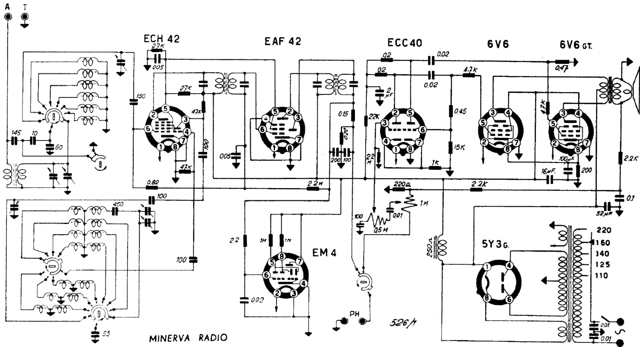
MINERVA RADIO - Mod. Viareggio tipo 526/1. Supereterodina a 6 valvole. Onde medie da 190 a 580 m. Corte con 6 espansioni di gamma: 49, 41, 31, 25, 19, 17 m. Media frequenza 468 kc. Potenza d'uscita 8 W. Consumo 80 W.
